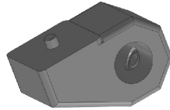
Kamerahalter mit 1/4'' Kameragewinde
